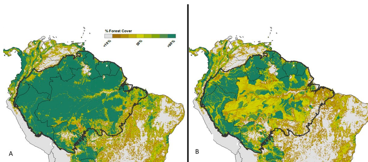
Figura 5. Desmatamento projetado do presente até 2050. Cobertura florestal do modelo para o presente (A - painel esquerdo) e 2050 (B - painel direito). A área de estudo do modelo é mostrada com uma linha escura. Espera-se que o contágio aumente com a perda de cobertura florestal e aumento da área de borda de floresta.
