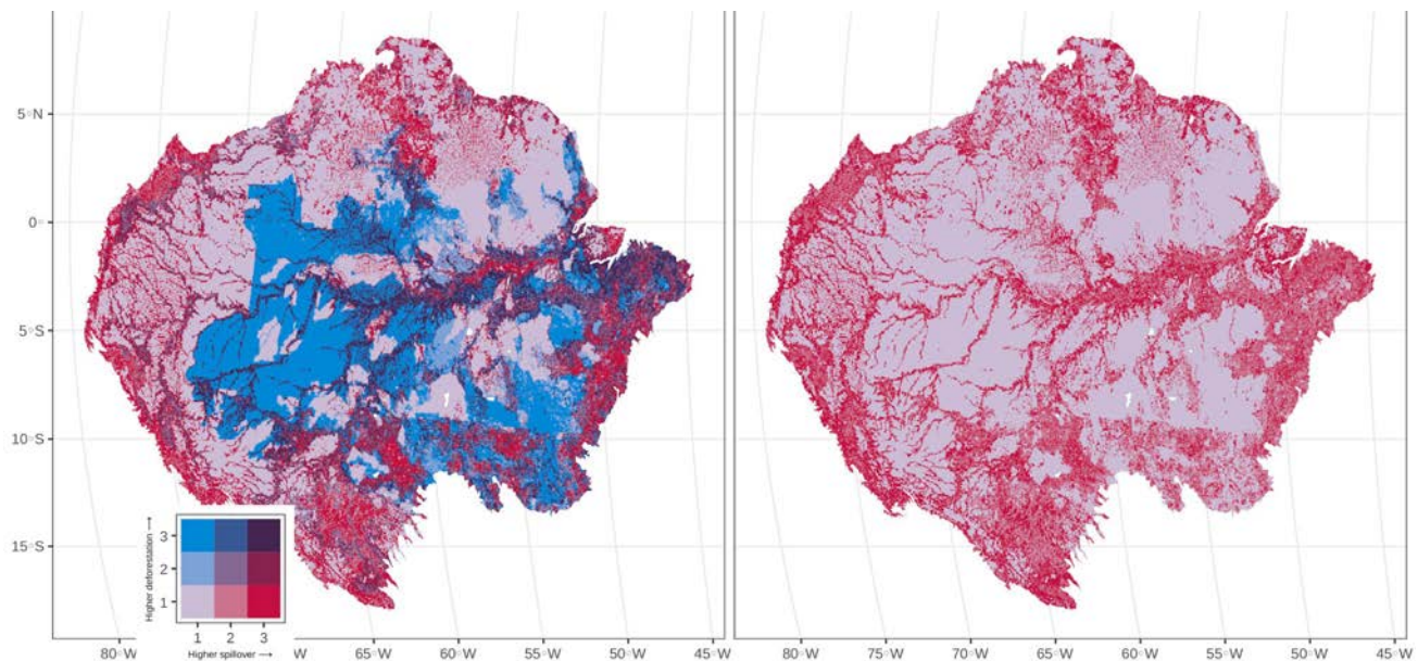
Figura 7. Mapa da Amazônia (linha branca) e número médio projetado de eventos de contágio per capita e alteração da cobertura entre 2020 e 2050 (desmatamento). Áreas que atualmente têm uma alta cobertura florestal (maior que 60%) e sofrerão baixo desmatamento terão baixos níveis de contágio (menor que 0,12, célula do canto inferior esquerdo no código de cores) e devem ser protegidas contra o desmatamento. Áreas de elevado contágio e alto desmatamento concentram-se em torno de centros populacionais e devem ser priorizadas no planejamento de uso da terra e apoio à saúde. Muitas áreas na Amazônia já estão desmatadas e terão um alto nível de contágio (maior que 0,3), mesmo que sofram pouco desmatamento adicional (menor que 40%) até 2050 (célula do canto inferior direito no painel de código de cores inserido). Essas áreas devem ser consideradas em programas de restauração, como o Plano de Recuperação de Vegetação Nativa (PLANAVEG-Brasil).
